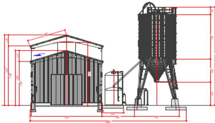
Neue Salzhalle Straßenmeisterei Tettnang Seitenansicht
